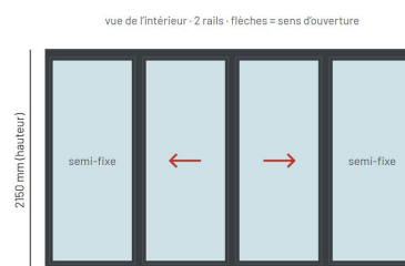
Coulissant 4 vantaux, ouverture au centre
